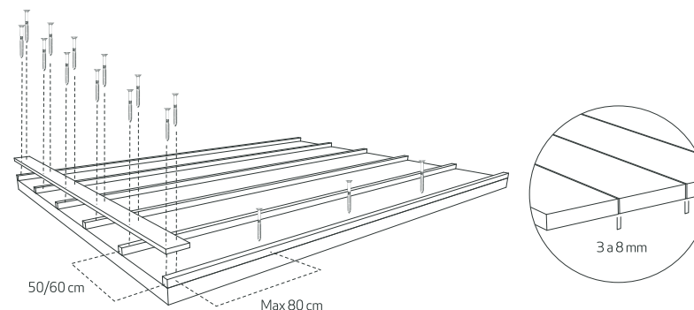
DESENHO TÉCNICO
