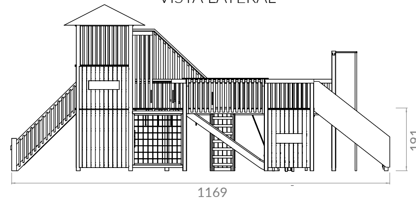
VISTA LATERAL
