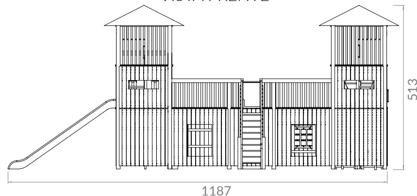
VISTA LATERAL
