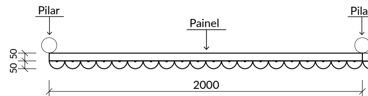
VISTA SUPERIOR
