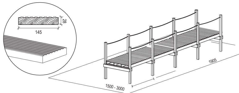
ALÇADO LONGITUDINAL
