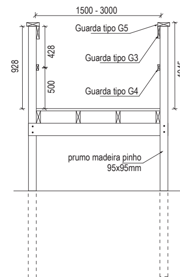
CORTE TRANSVERSAL
