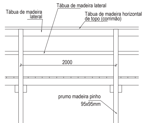
ALÇADO LONGITUDINAL
