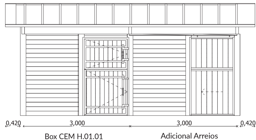
ALÇADO FRONTAL
