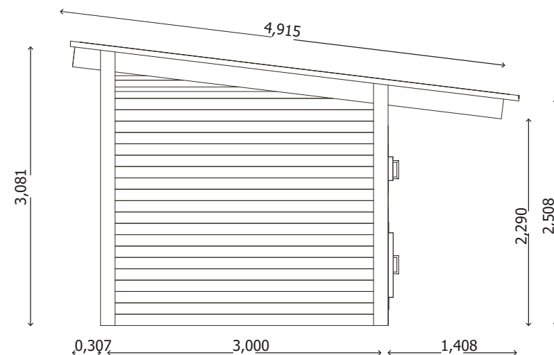
ALÇADO LATERAL
